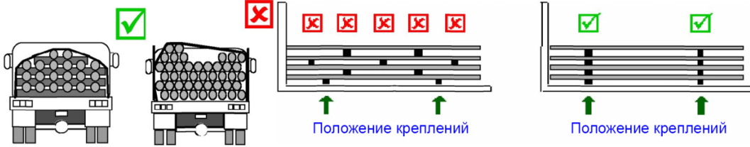
Крепление длинных труб с помощью амортизационных материалов
