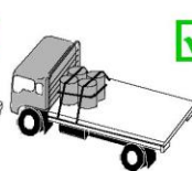
Сочетание стяжных ремней и прямого ограничения конструкции транспортного средства
