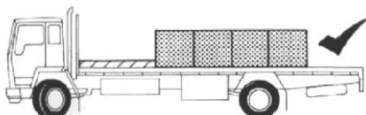
Размещайте грузы дальше назад для лучшего распределения нагрузки и поддерживайте центр массы как можно ниже.
