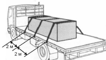
СТЯЖНЫЕ РЕМНИ
