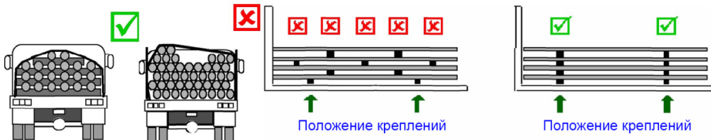
Крепление длинных труб с помощью амортизационных материалов
