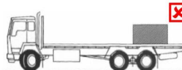
Размещайте центр массы груза перед центром задней оси (группы)
