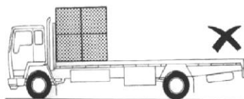
НЕПРАВИЛЬНОЕ ПОЛОЖЕНИЕ ГРУЗА (перегрузка передней оси)
